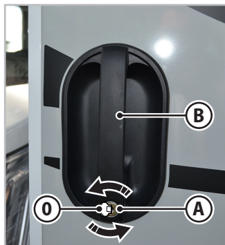
Εικ.5.1 - Άνοιγμα/κλείσιμο της πόρτας εισόδου από έξω
