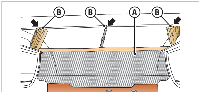
Εικ.6.18 - Δίκτυ ασφαλείας πτυσσόμενου κρεβατιού
