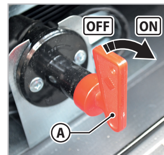
Εικ.6.30 - Διακόπτης αποσύνδεσης μπαταρίας
