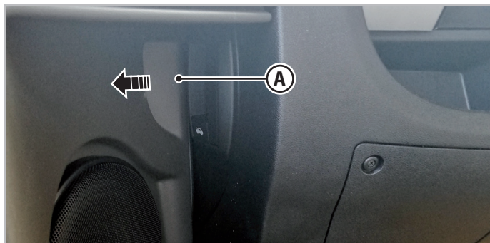
Εικ.5.8 - Μοχλός ανοίγματος καπό - Τύπος A
