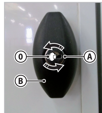
Εικ.5.4 - Άνοιγμα/κλείσιμο χώρου γκαράζ
