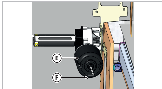
Εικ.6.17 - Ηλεκτρικό ξεκλείδωμα κρεβατιού τύπου Β
