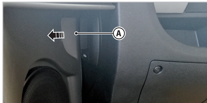
Fig.5.8 - Greb til åbning af motorhjelms - Type A
