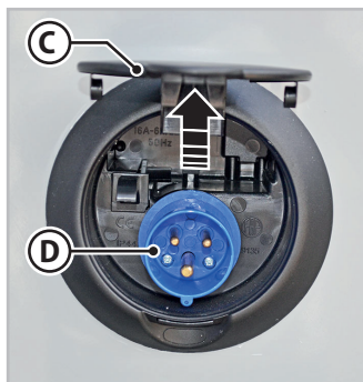
Fig.6.29 - 220 V stikkontakt
