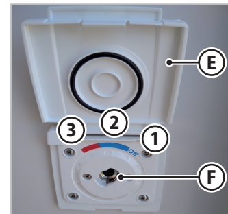
Фиг.6.34 - Конектор за свързване на душа
