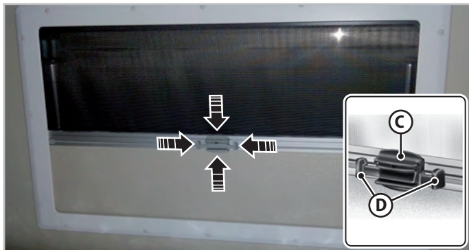
Фиг.6.4 - Мрежа против комари и затъмняваща щора на прозореца
